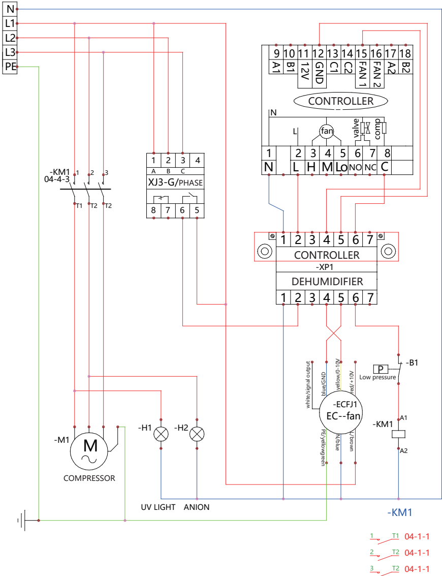
FD-S180/250L-DEHUMIDIFIER WIRING DIAGRAM
